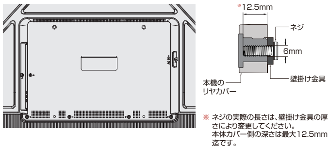
壁掛け用ネジ穴 (VESA規格) 4-M6(深さ12.5mm)
